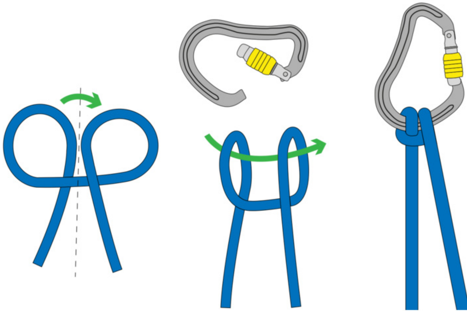
Munter Hitch
